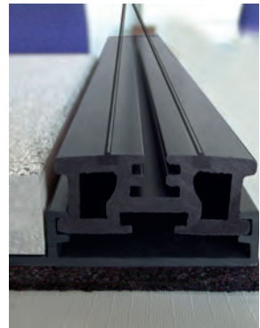
Montage auf abgedichteten Flächen
